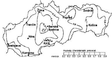
ODHAD PRESNOSTI ROČNÝCH RÝCHLOSTÍ RECENTNÝCH POHYBOV
