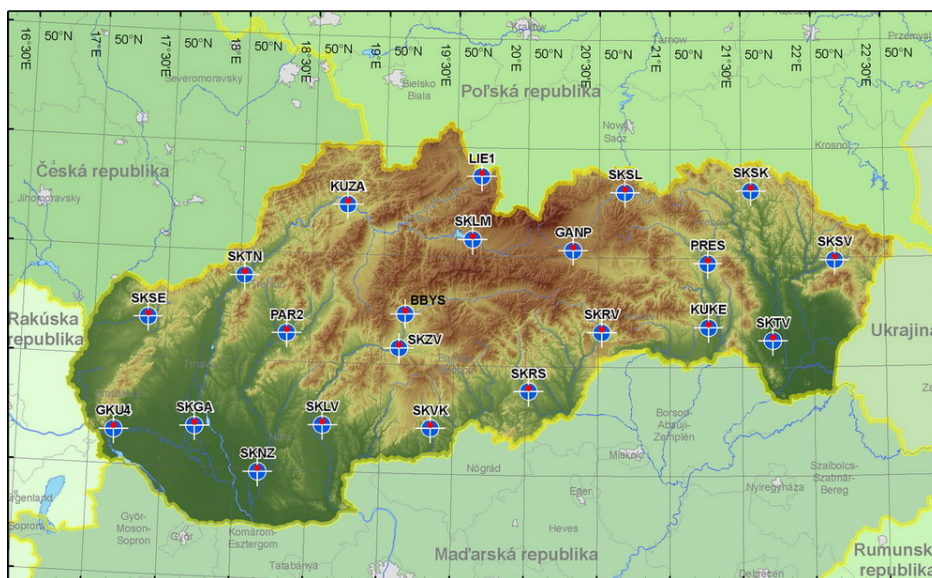
Obr. 1 Schéma staníc SKPOS
