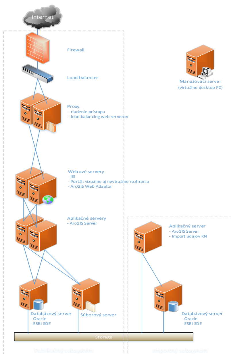
Diagram č. 2: Serverová architektúra riešenia
