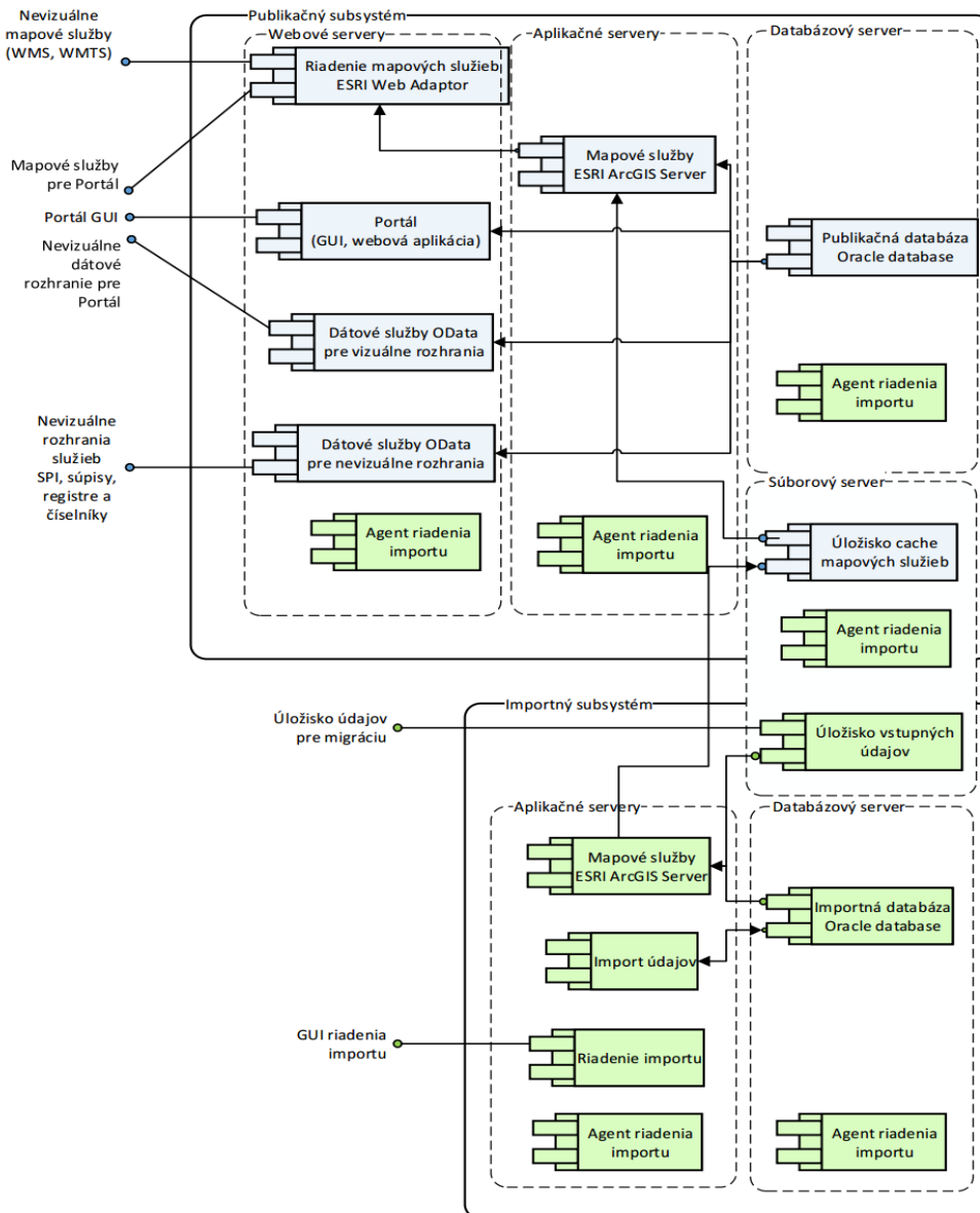
Diagram č.1: Komponentná architektúra riešenia
